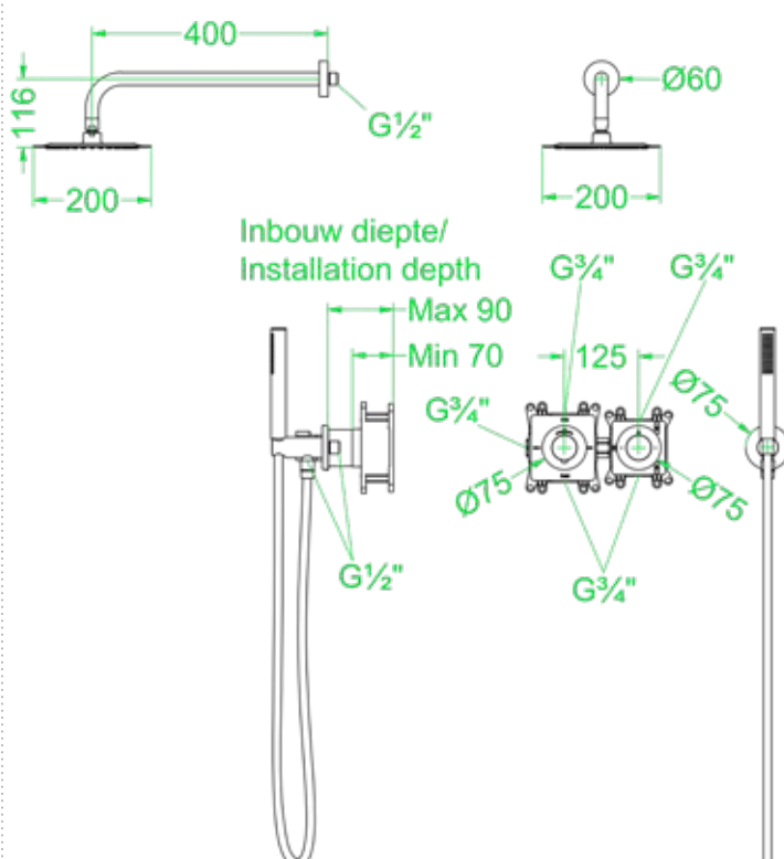
Pact afbouwdeel inbouwthermostaat met 2-weg stop-omstel Pact external part of concealed thermostat with 2-way stop-diverter
